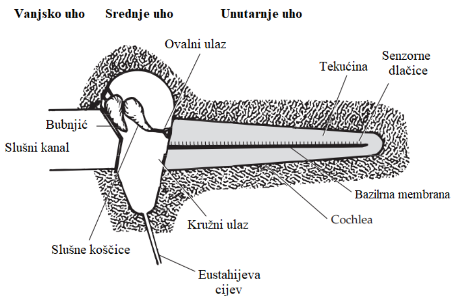
Slika 14: Prikaz ljudskog uha s „odmotanom“ pužnicom (Izvor: Everest i Pohlmann, 2009, str. 44)
