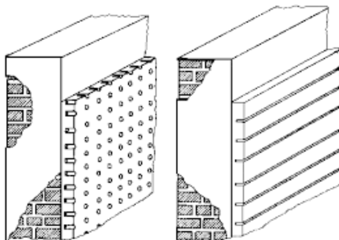
Slika 40: Rezonatorski apsorberi
