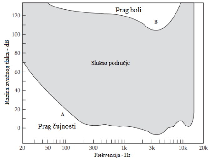
Slika 16: Slušno područje (osjenčano područje), prag čujnosti (krivulja A) i prag boli (krivulja B) (Izvor: Everest i Pohlmann, 2009, str. 48)
