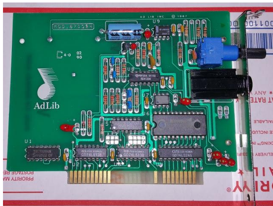
Slika 13. AdLib zvučna kartica
